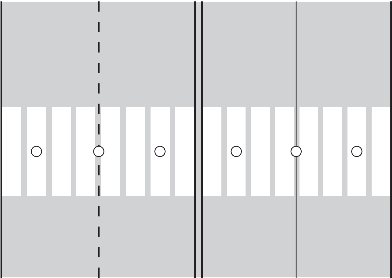
4 Corsie - disposizione a una stringa centrale - GECO PULSE 9K (luce lampeggiante) - art. GECO-P-9K-CR
